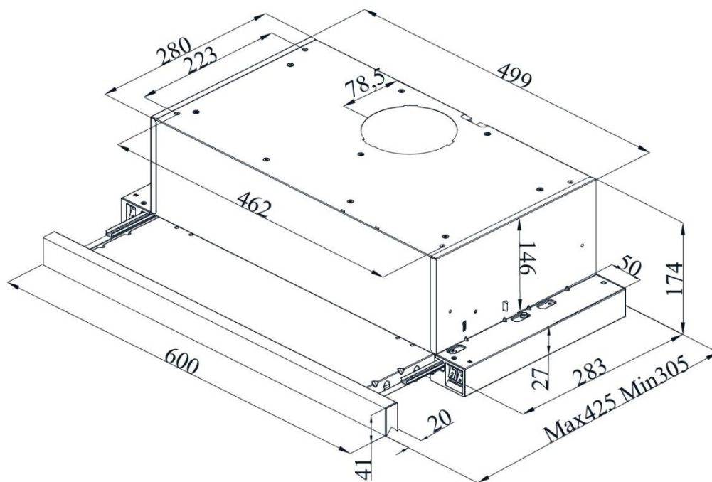
1. ábra 1350 beépítési rajz
