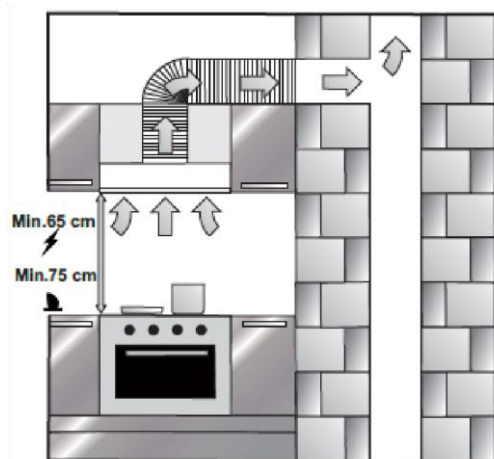
8. ábra Minimum és maximum beszerelési méretek
