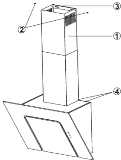
13. ábra kürtő takaró elemek összeszerelése
