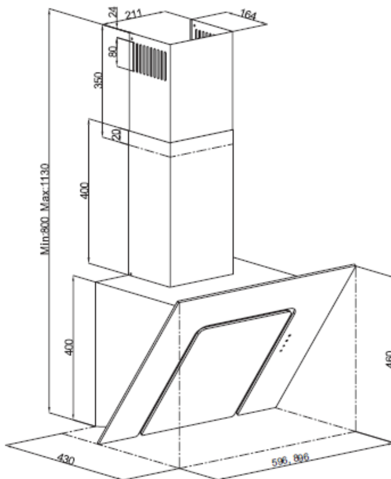
1. ábra 3423 méretezett beépítési rajz
