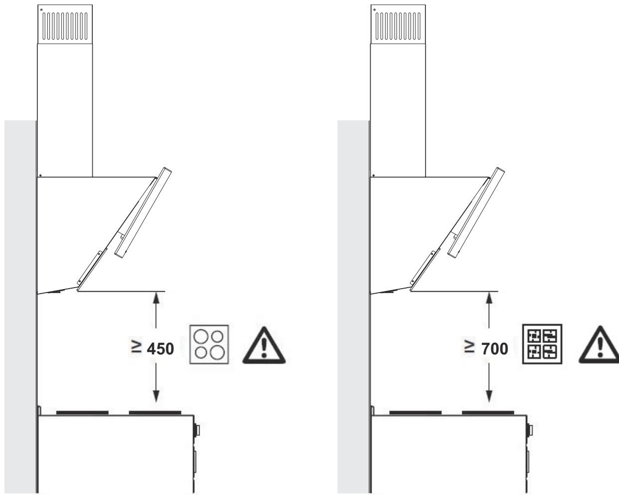
Fig. 8: Montering/Installation af produktet
