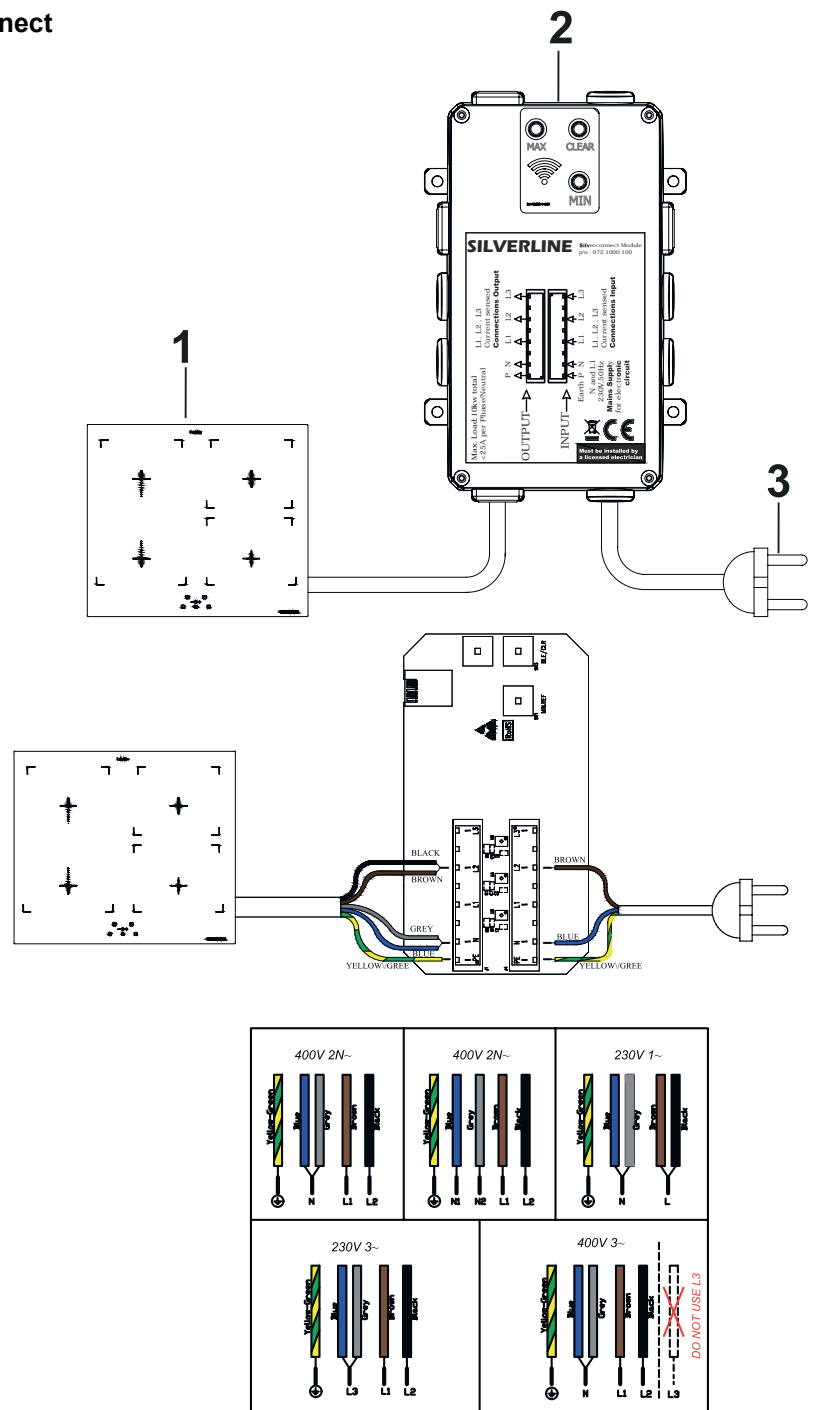
Fig. 27: Anslutning av spishäll och SilverConnect
