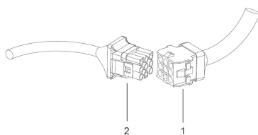
Fig. 29: Multistik forbindelse
