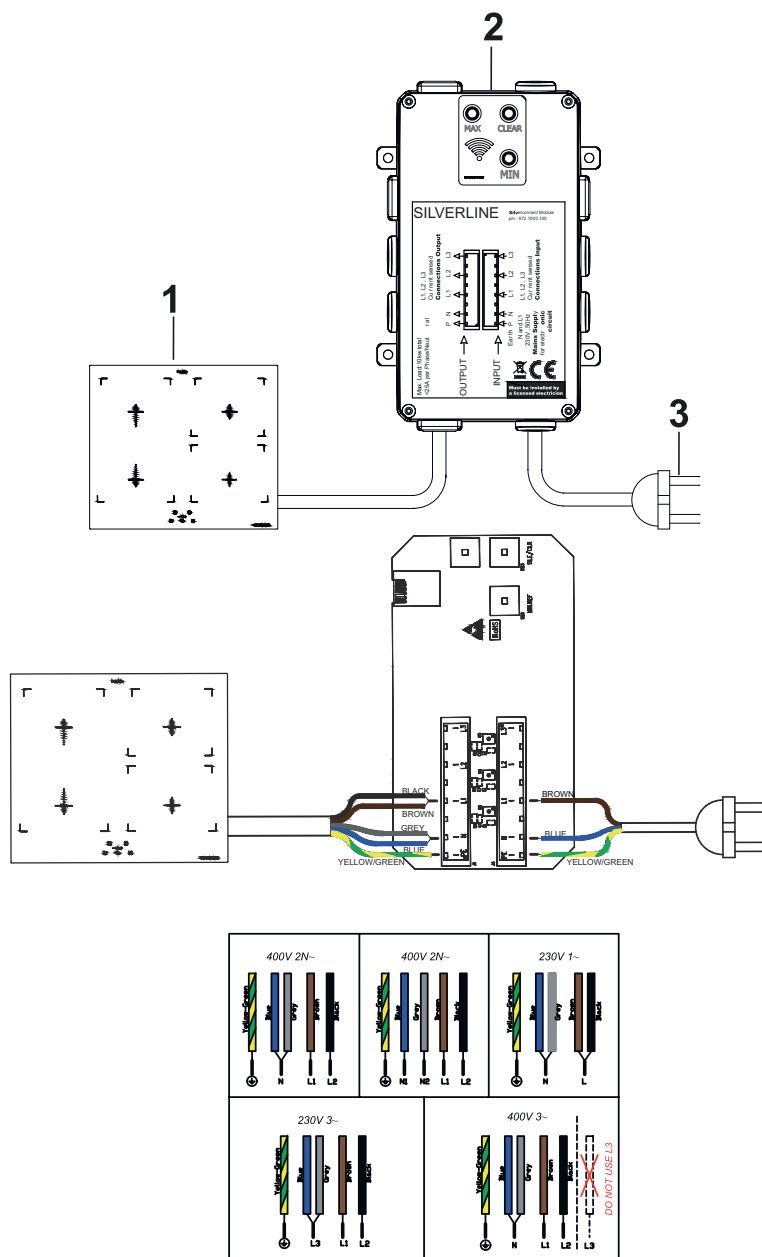
Fig. 24: Forbindelse af kogeplade og silverconnect
