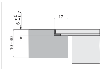
Fig. 18: Mål bruges i forbindelse med planlimning
