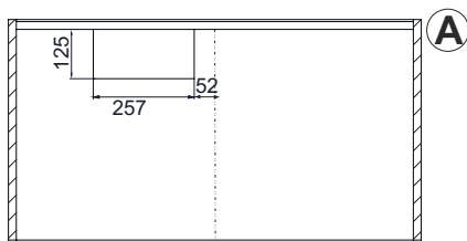
Fig. 21: Eksempel på montering
