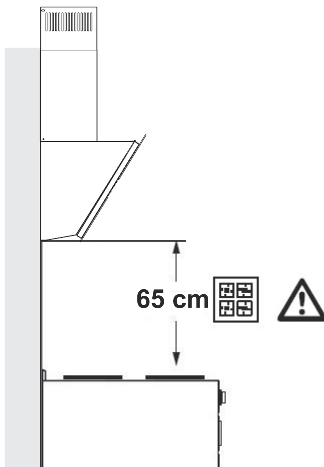
Fig. 15: Montering/Installation af produktet
